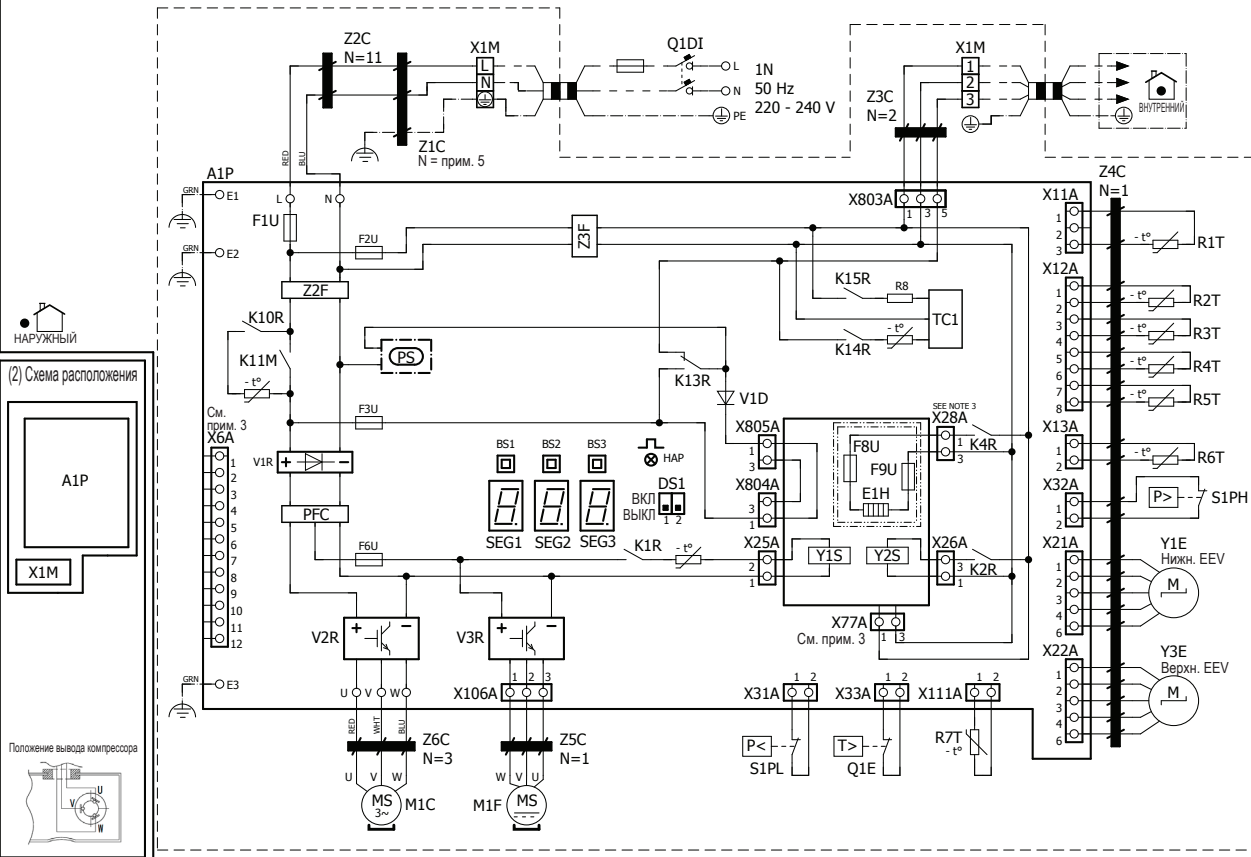
(1) Схема соединений
