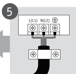
5 Подсоедините кабели
