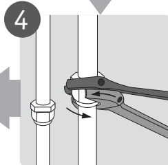
4 Присоедините трубы хладагента
