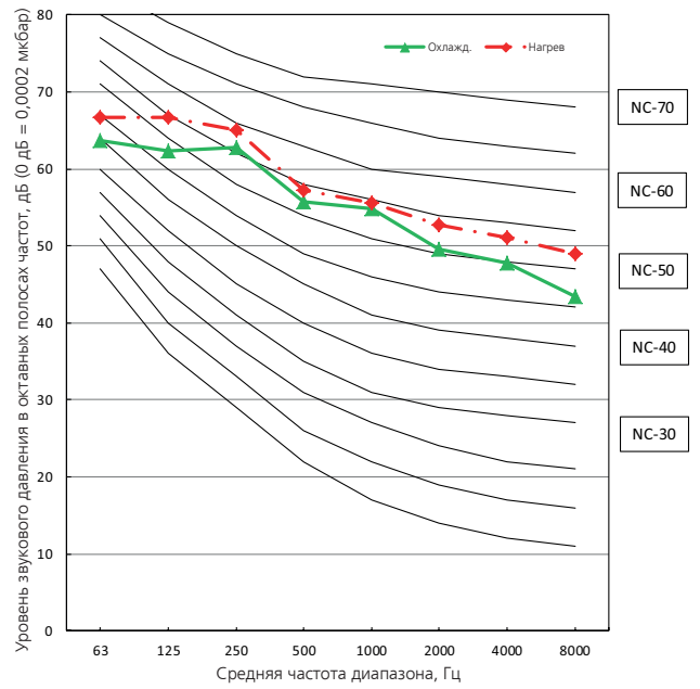
M4OB-36HFN8-Q1
