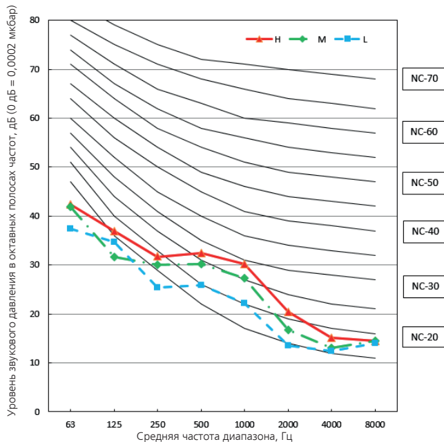
MTIU-12HWFNXP(GA)
