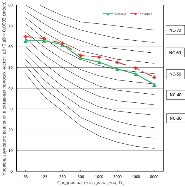
M4OE-28HFN8-Q1
