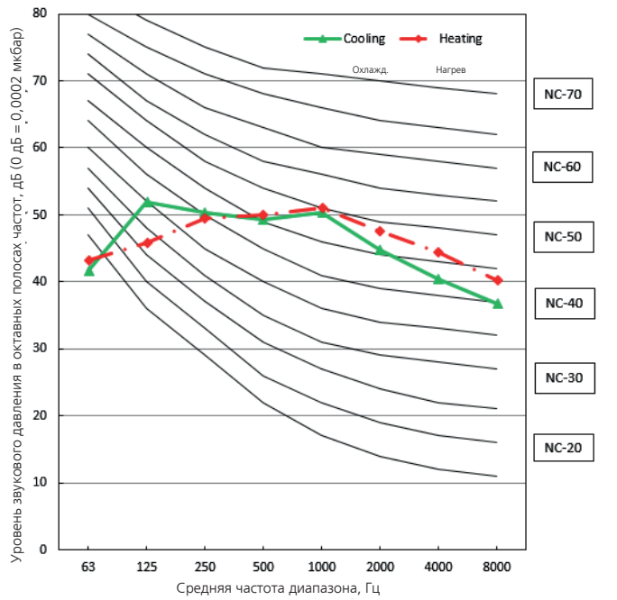
M3OA-27HFN8-Q1
