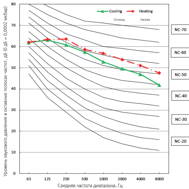
M5OE-42HFN8-Q1
