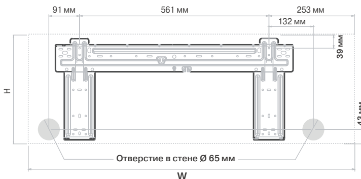
Отверстие в стене \varnothing 65 мм Размеры внутреннего блока (Ш×В): 968 мм x 322 мм
