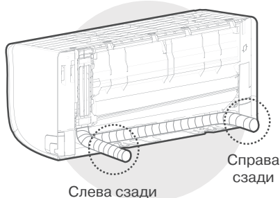
Четыре варианта вывода трубопровода
