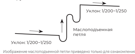
Изображение маслоподъемной петли приведено только для ознакомления
