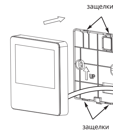
защелки
